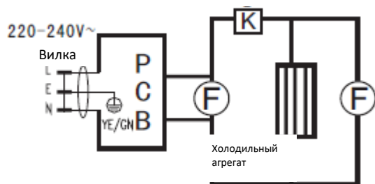
Электрическая схема
