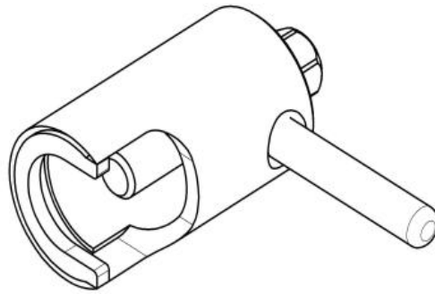
Рис. 13. Съемник крыльчатки.
