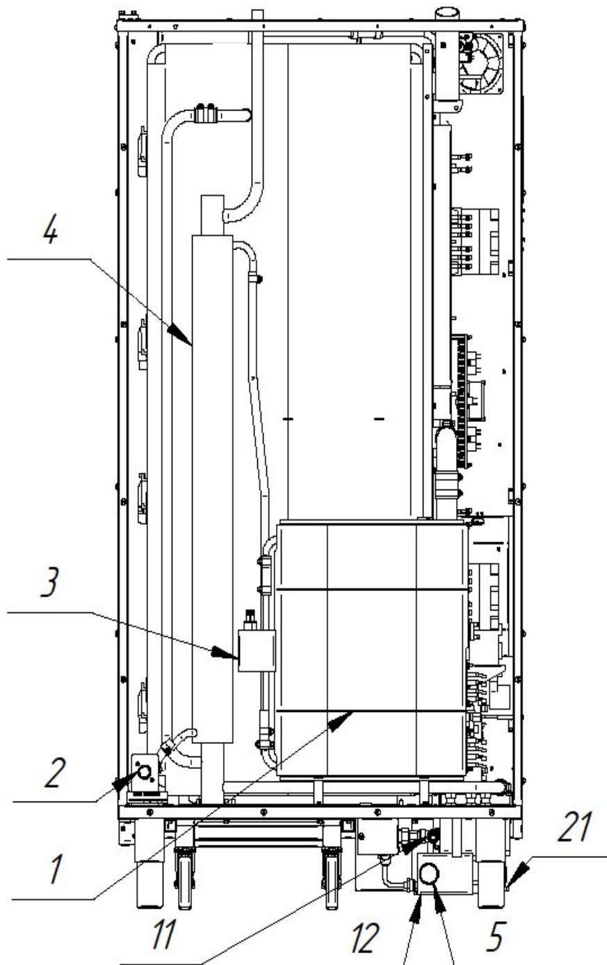
Рис.2а. Система водоснабжения, водоотведения и автоматической мойки (вид сзади)
