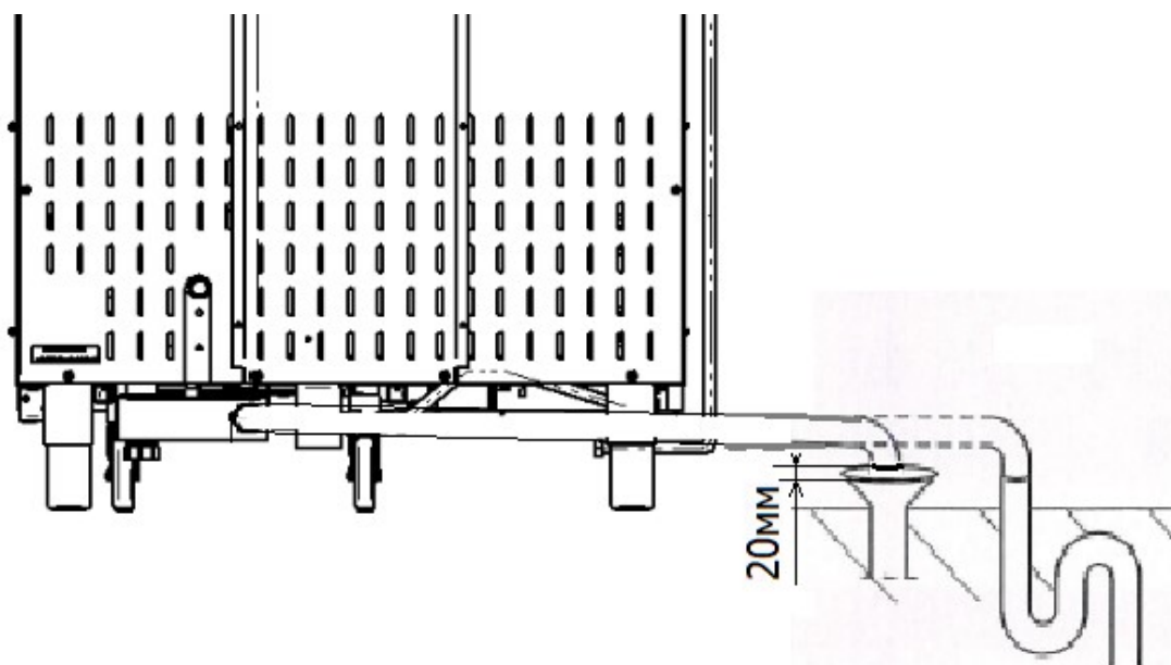
Рис. 9 Подключение пароконвектомуата к канализации с разрывом струи.
