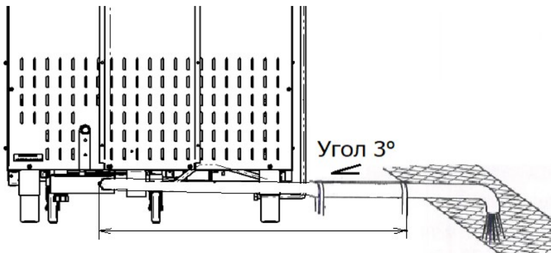
Рис. 8 Подключение пароконвектомуата к канализации – слив в трап.
