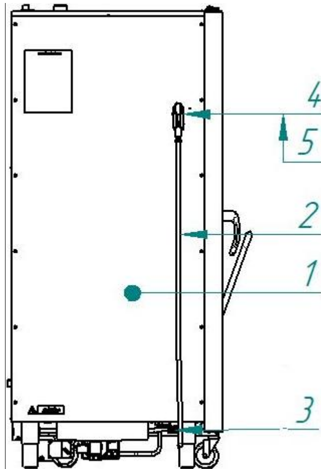
Рис. 10 Подключение пароконвектомата к канализации – слив в пол (разрыв струи).
