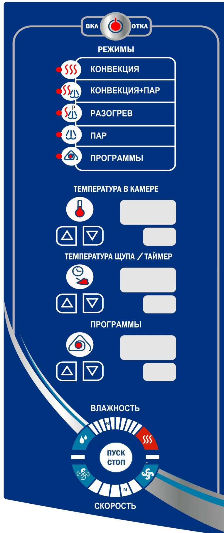
Рис. 3. Пленочная клавиатура
